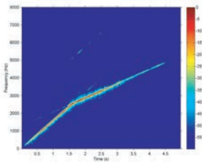
소리 왜곡을 최소화한 리사운드의 주파수 압축방식
