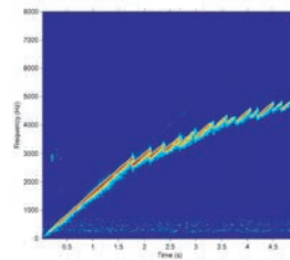
타사 주파수 압축방식의 소리 왜곡
